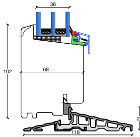
D3: Dørtrin indadgående dør (kan leveres med dobbelt spændestykke)
