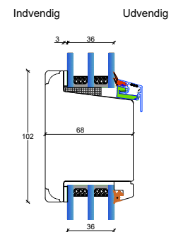
105 mm. gennemgående sprosse Modern
