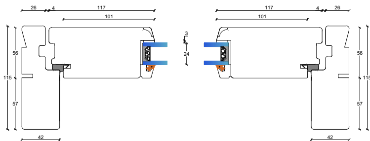
D2: Topkarme døre, udadgående
